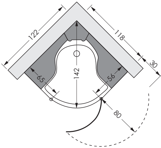
Draufsicht, Abb. Anschlag rechts
