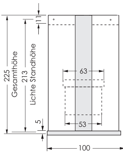
Standardhöhe, Abb. U-Version, Anschlag links
