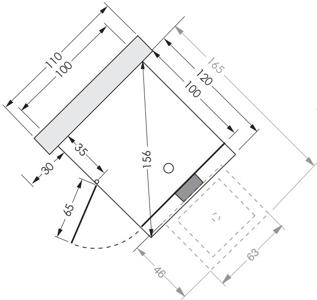
Draufsicht U-Version, Abb. Anschlag links
