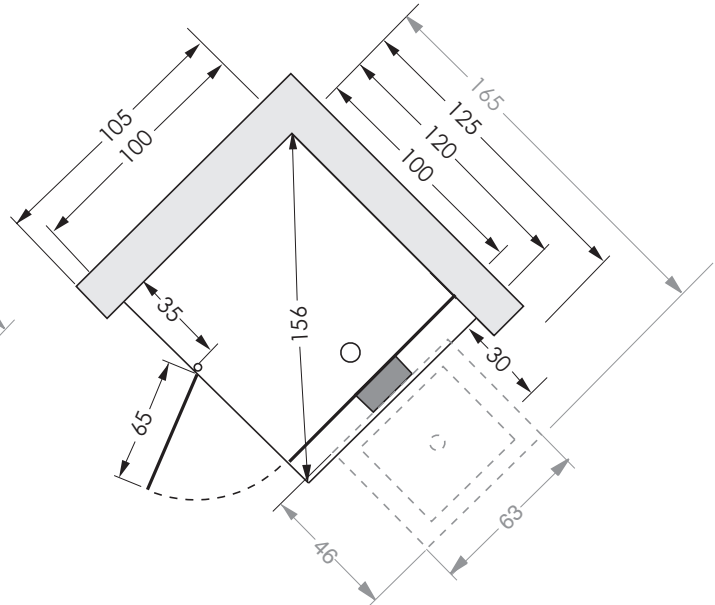
Draufsicht Eck-Version, Abb. Anschlag links, Sitz links
